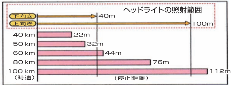
図3 ヘッドライトの照射範囲と車の停止距離※
